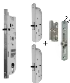
Serrure automatique SAM 5 points «à enclenchement soft»: - avec 3 pénes - 2 galets champignon + gâches antiécartement - enclenchement automatique des 3 pénes en douceur - verrouillage des 2 galets par manoeuvre à la clé
