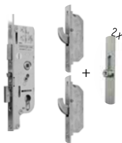
Serrure automatique SAC 5 points à crochets «sécurité +»: - avec 2 crochets, 1 pêne central et 2 rouleaux à déclenchement automatique
